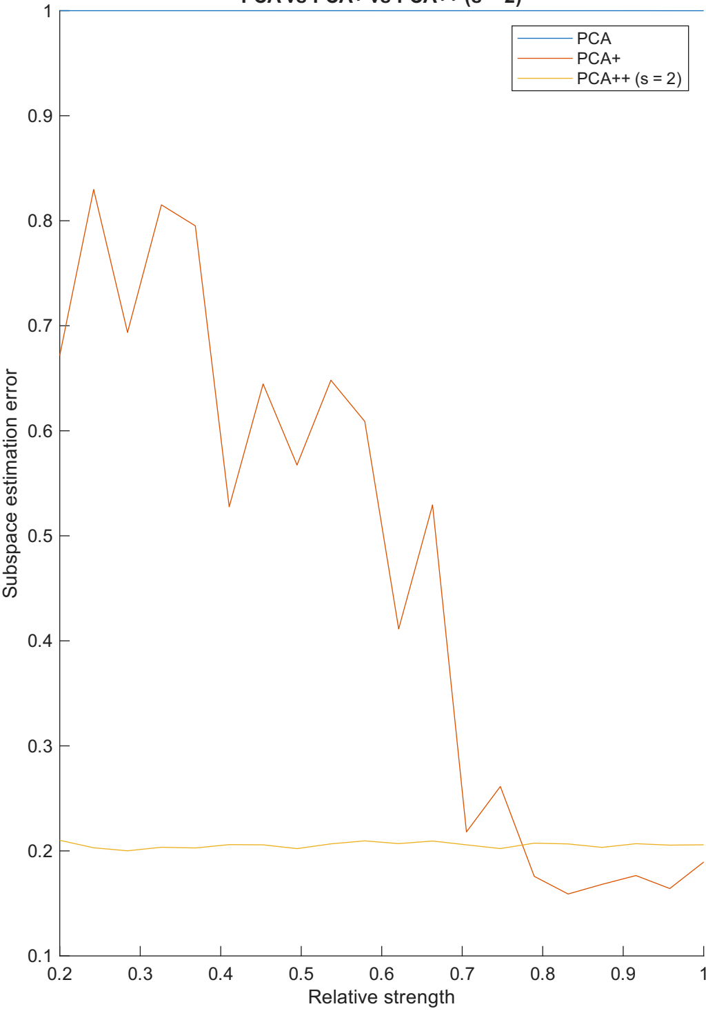
PCA vs PCA+ vs PCA++ (s = 2)
