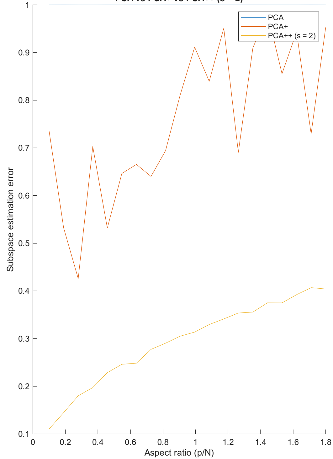
PCA vs PCA+ vs PCA++ (s = 2)
